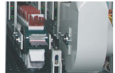
Spazzola trasversale - Cross brush - Quer Bürste
